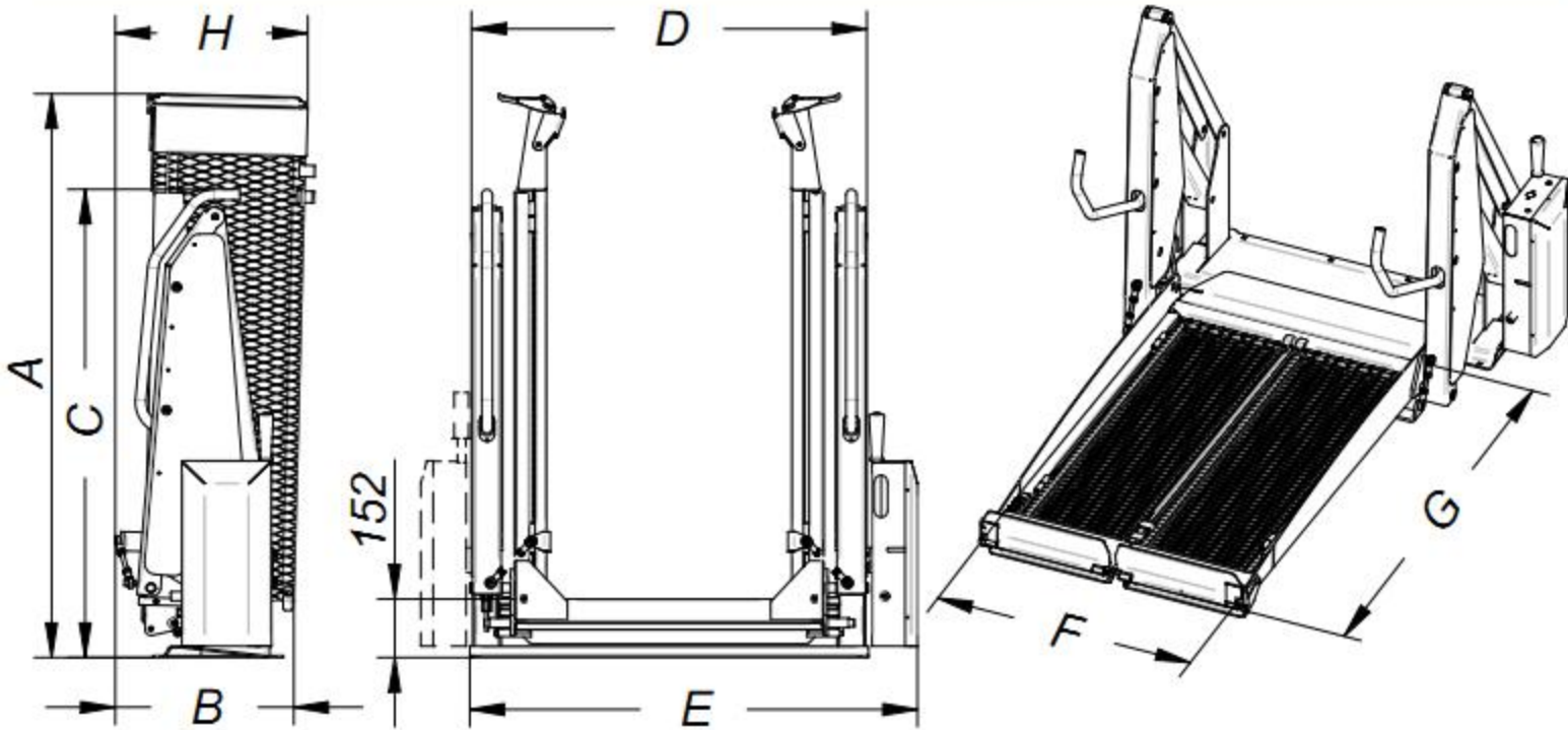
Габаритные размеры
