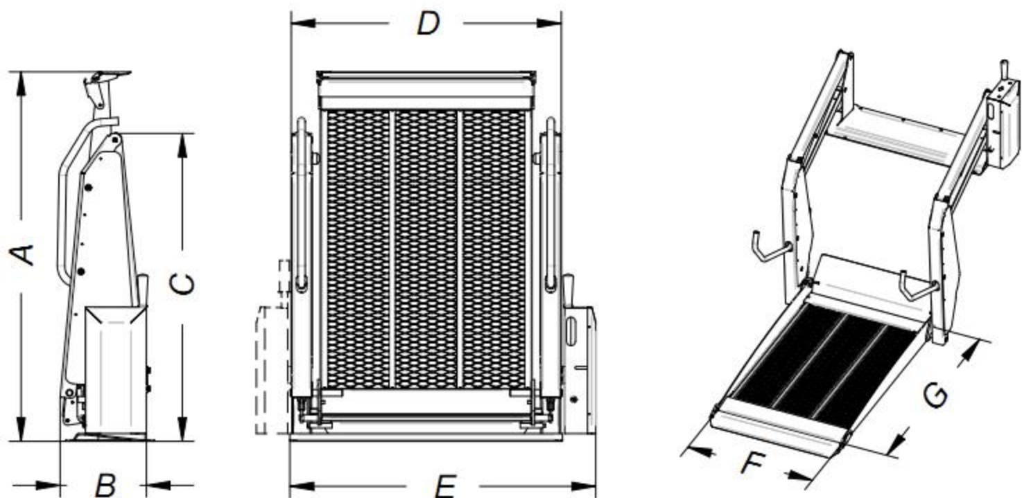
Габаритные размеры
